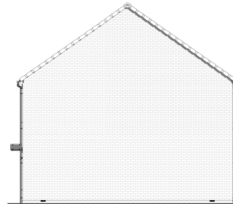
RIGHT ELEVATION 1 : 100
