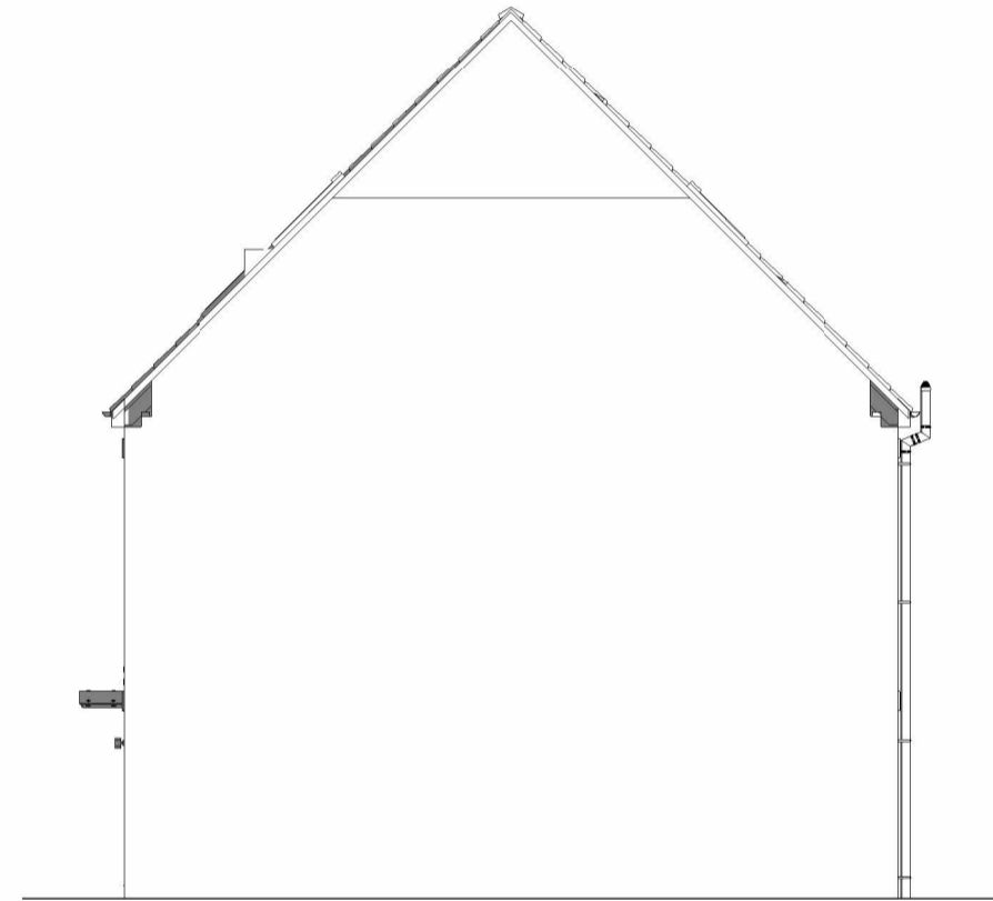
RIGHT ELEVATION 1 : 100
